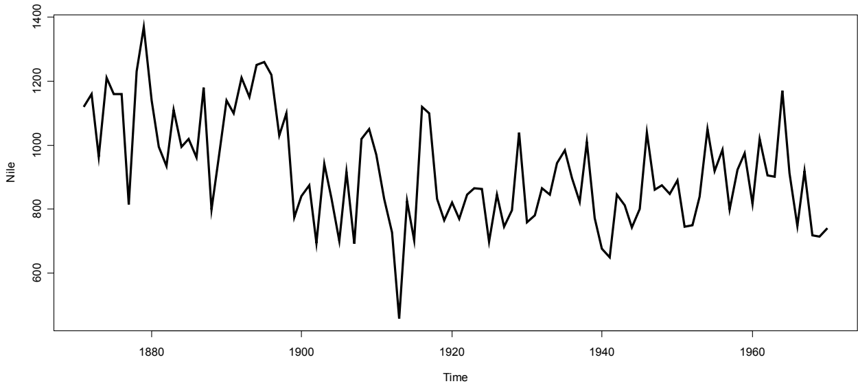
Débit du Nil 1871-1970
